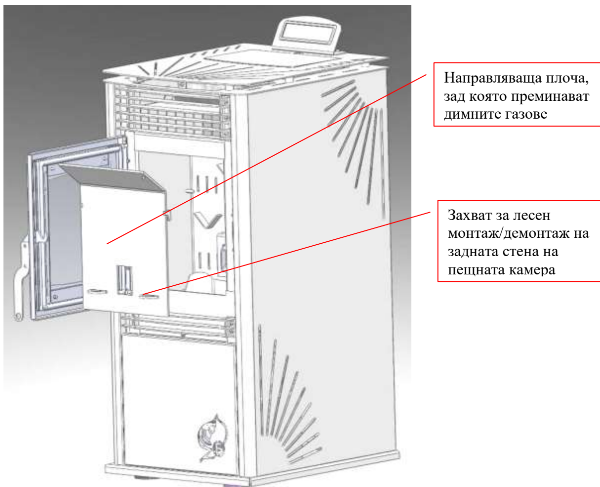
Фигура 5.4. Изглед на автоматизираната топовъздушна камина, оползотворяваща пелети от серията “Рору” с отворена врата и демонтирана направляваща (димните газове) плоча;
